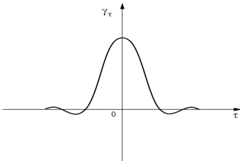
Figura 2.3: Função de autocovariância
