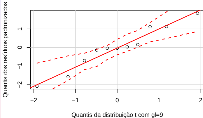
Figura 9: Gráfico QQ correspondente ajuste do modelo de regressão linear aos dados da Tabela 1 (sem a observação influente).
