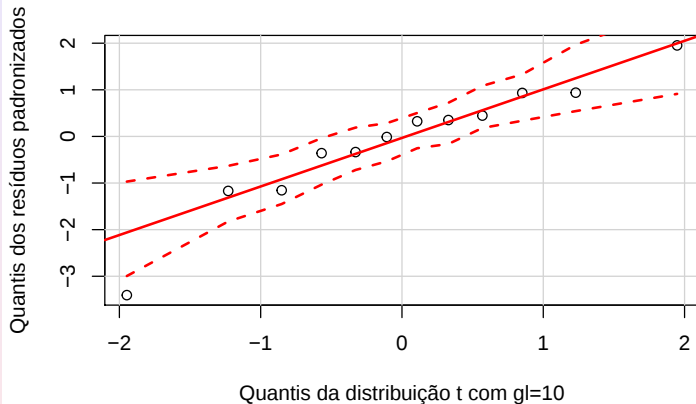
Figura 8: Gráfico QQ correspondente ajuste do modelo de regressão linear aos dados da Tabela 1 (com todas as observações).
