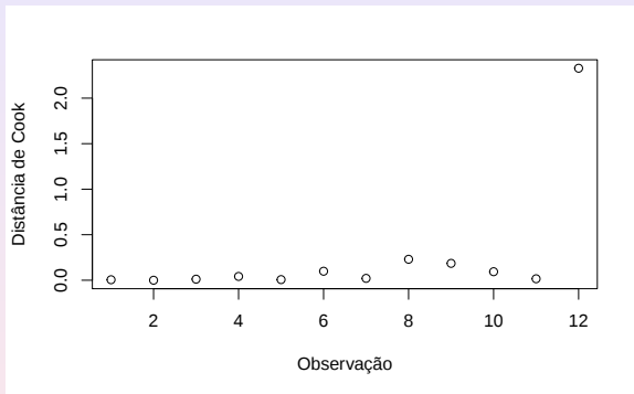
Figura 6: Gráfico de Cook correspondente ao ajuste do modelo de regressão linear aos dados da Tabela 1.
